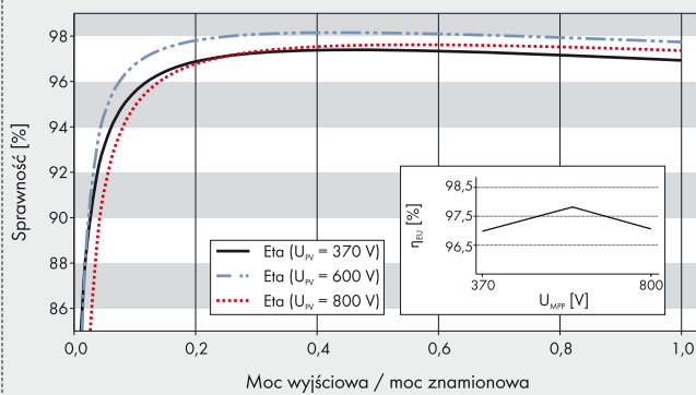
Wykres sprawności SUNNY TRIPOWER 9000TL
